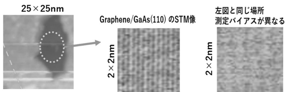
Fig.2 Graphene/GaAs (110) の STM 像。暗い領域の拡大図が中央。同じ場所を条件を変えて測定した画像が右図。
