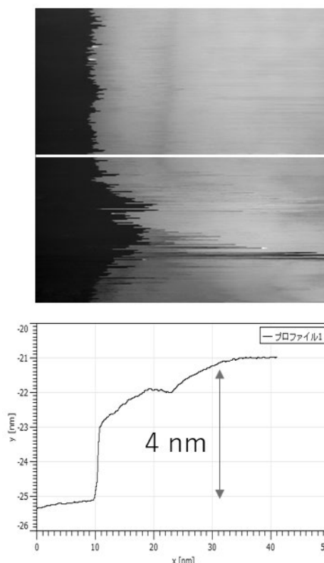
Fig.1 40nm 四方 STM 像 GaAs(110) 上の Gr までの段差
