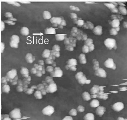
Fig.5 400×400nm GaAs-0.3ML 成長後の Gr./ GaAs 表面 STM 像
